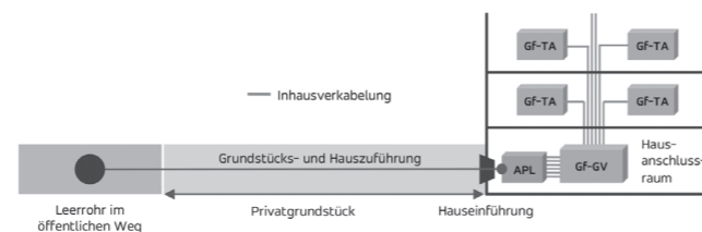
Prinzipiskizze Mehrfamilienhaus
