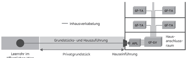
Prinzipiskizze Mehrfamilienhaus
