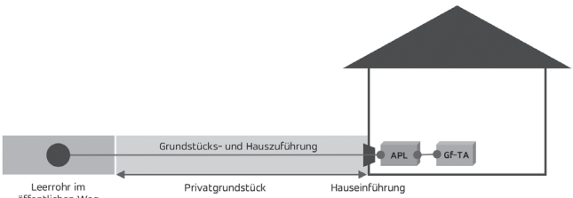
Prinzipiskizze Ein- und Zweifamilienhaus
