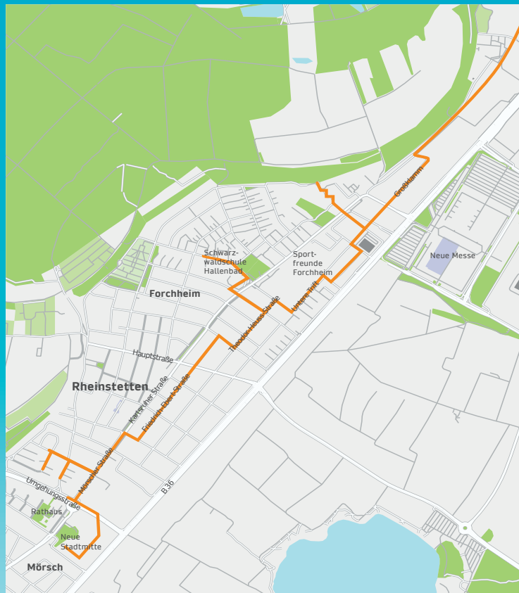
Fernwärme-Netzplan
